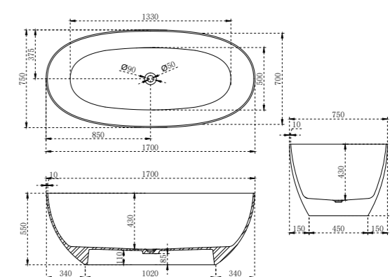
VBT-6T01B Размеры, мм: 1700x750x550
