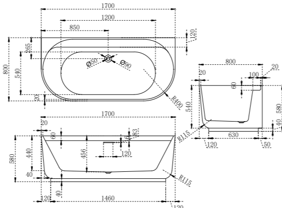
VBT-621B Размеры, мм: 1700x800x580
