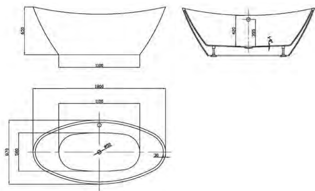
VBT-203 Размеры, мм: 1800x870x650
