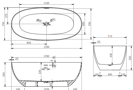
VBT-6S01 Размеры, мм: 1700x720x550
